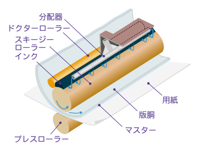
最適な量のインクを均一に移転させる、印刷ドラムの多層構造
