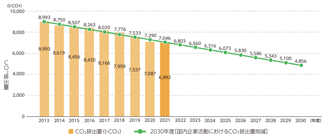
図表 2 国内企業活動における CO 2 排出量の推移
